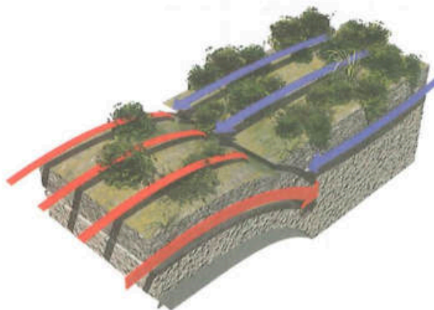
Interacciones de placas tectónicas
