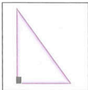
Triángulo rectángulo
