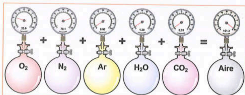
▲ Utilizando el aire, que es una mezcla de gases, se puede explicar la ley de las presiones parciales.
