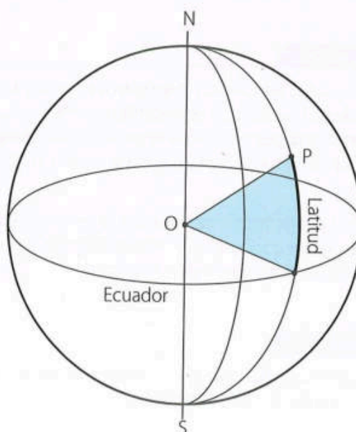
▲ La parte sombreada corresponde a un arco de un meridiano, valor tomado en cuenta desde la línea ecuatorial hacia la latitud norte, en este caso.
