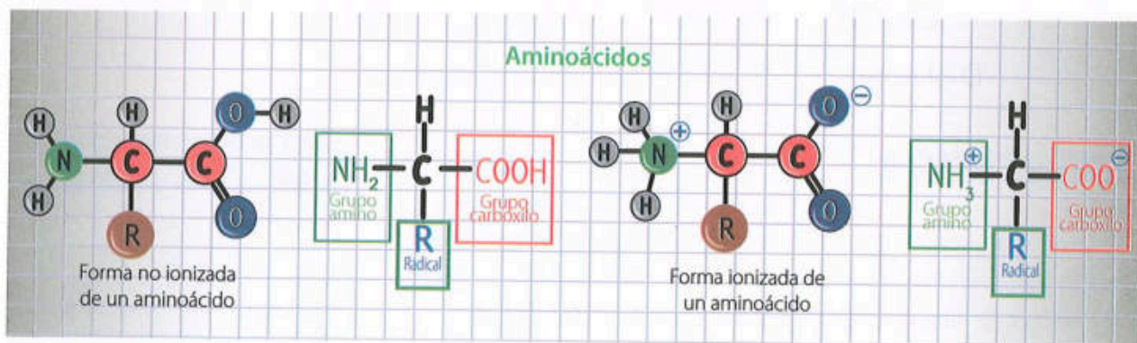
▲ Representación de la estructura general de un aminoácido: se identifica el grupo carboxilo y el grupo amino.
